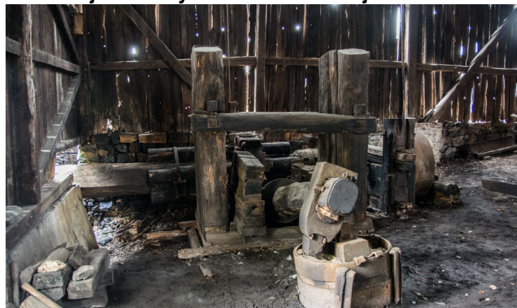
Drewniany młot naciskowy w Starej Kuźnicy
